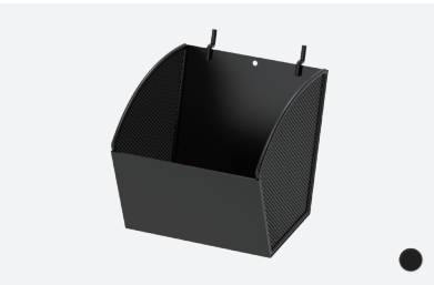
HH-T-07 Grid Box 12(L)x8(W)x11(H) cm 4.72"(L)x3.15"(W)x4.33"(H)
